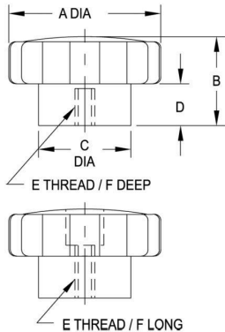
1/4-20 CL-340-PFK 5/16-18 CL-350-PFK
